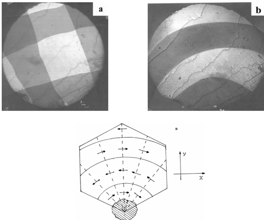
1 - rasm. «Yelimlangan» \text{FeBO}_3 kristalli domenli strukturasining kuchlanganlik N=0 boʻlganda olingan tasviri: a) T=290 K va b) T=90 K; v –kuchlanganlikka ega boʻlgan kristall bazisli tekisligidagi spontan magnitlanish (strelkalar) vektorining fazoviy taqsimoti. Punktir chiziqlar mexanik kuchlanish taʼsir etuvchi yoʻnalishlar, shtrixlangan soha kristall ushlagichga mahkamlangan kley tomchisi. Oʻngda-laboratoriya koordinatalar sistemasidagi oʻqlar yoʻnalishi: X oʻqi S_2 ning uchta oʻqidan bittasi bilan mos keladi, Z -oʻqining yoʻnalishi S_3 oʻqi yoʻnalishi bilan mos keladi [4,5].
