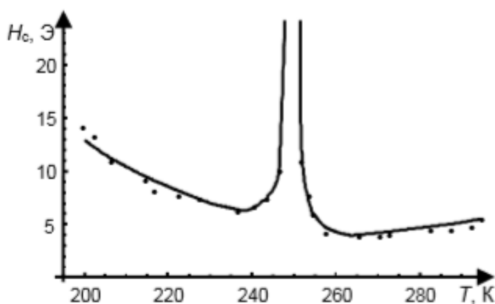
Рис.1. Температурная зависимость напряженности внешнего магнитного поля, при котором образец переходит в однодоменное (однородно намагниченное) состояние: сплошная линия – расчет по (4), точки – эксперимент.
