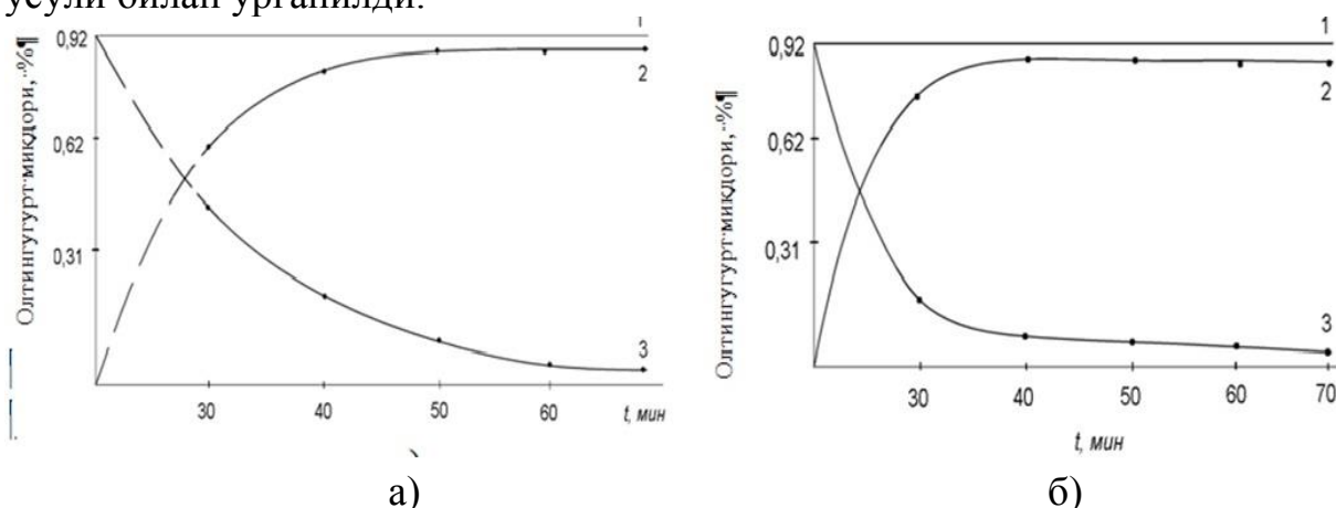
1-расм. SKMS-30APKM-15 (а) ва SKI-3 (б) асосидаги резина аралашмаларини вулканизациялаш вақтининг олтингурут бирикиши кинетикасига таъсири.
