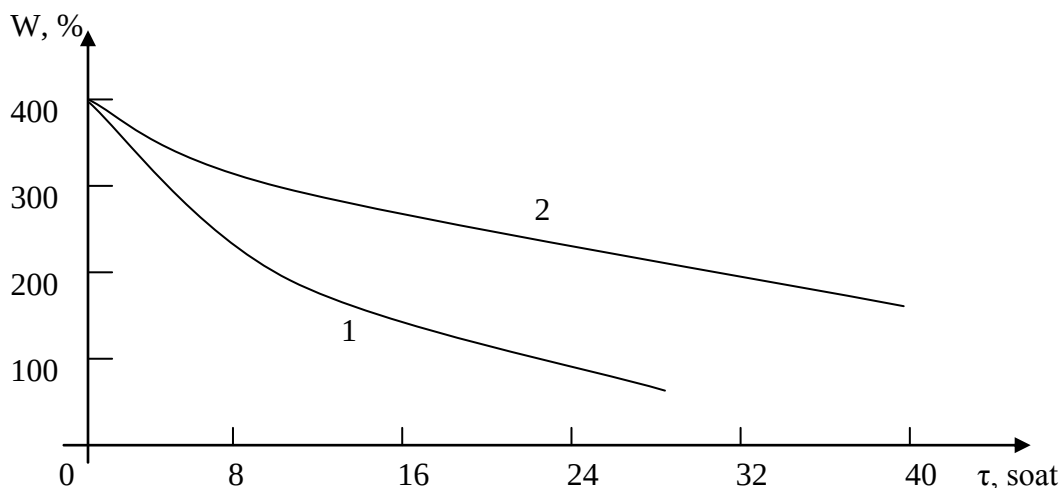
2-расм. Hermetia illucens личинкаларини куритигчада (1) ва очик ҳавода (2) қуриштиш натижалари.
