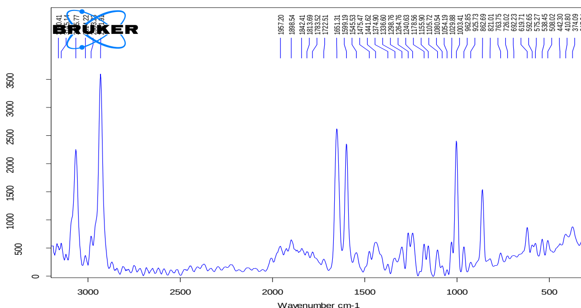
1-rasm. Atsetoatsetanilidning atsetil gidrazoni raman spektri
