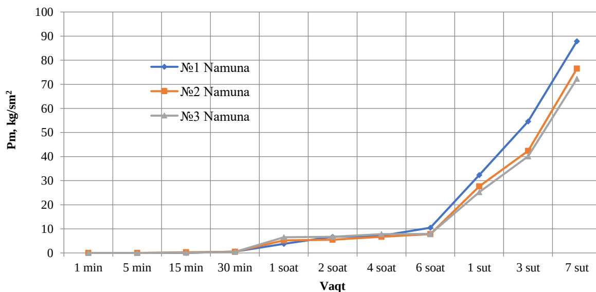
3 rasm. 700 ° C haroratda olingan gips bog'lovchilarining suspenziyalarida struktura hosil bo'lishining kinetikasi S/G 0,3
