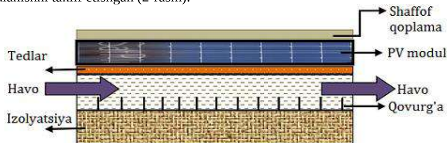
2-rasm. Modifikatsiyalangan havoli PVT tizim
