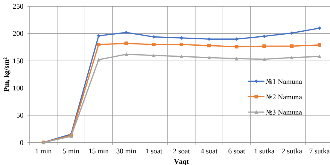
1 rasm. 160-180 °C haroratda olingan gips bog'lovchilarining suspenziyalarida struktura hosil bo'lishining kinetikasi S/G 0,5
