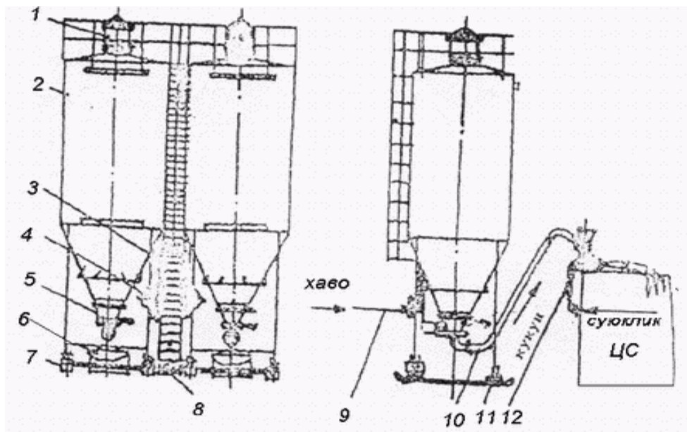
2-rasm. Burg'ilash eritmasini tayyorlaydigan ETQ -70 texnologik tizim qurilmasi.
