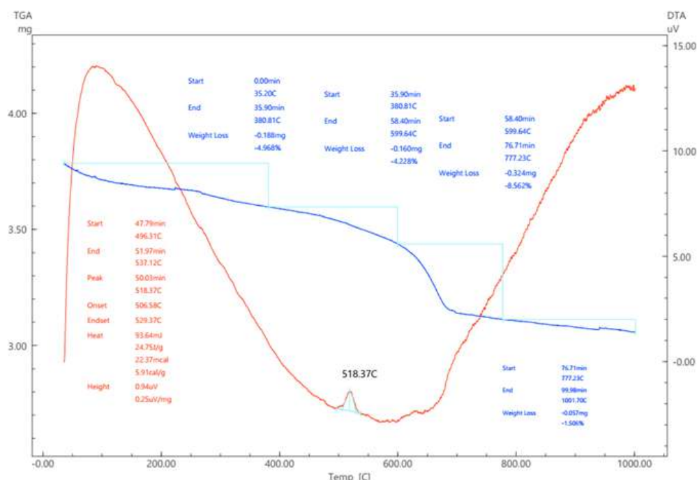
Рис.3 – Дифференциально-термический анализ (ДТА) Белтауской глины
