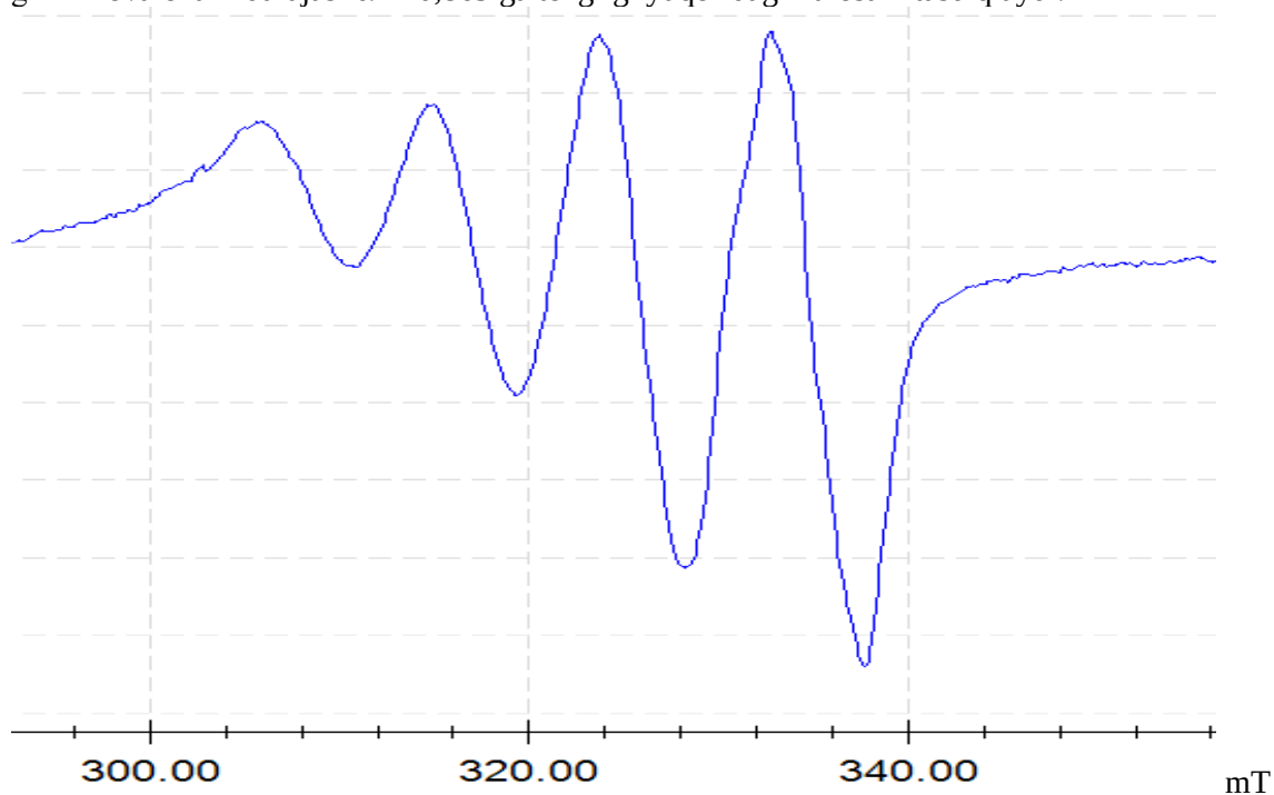
1-rasm. CuL \cdot NH_3 metanoldagi eritmasidan olingan EPR spektri
