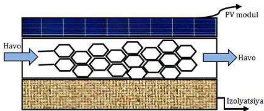
3-rasm. Uyali issiqlik almashinuv qurilmasi o'rnatilgan PVT tizim
