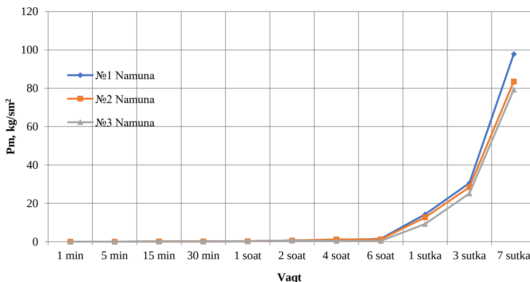
4 rasm. 1000 ° C haroratda olingan gips bog'lovchilarining suspenziyalarida struktura hosil bo'lishining kinetikasi S/G 0,3
