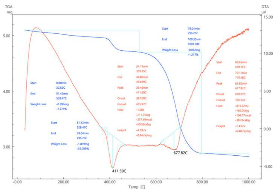
Рис.2 – Дифференциально-термический анализ (ДТА) отхода Кунградского содового завода
