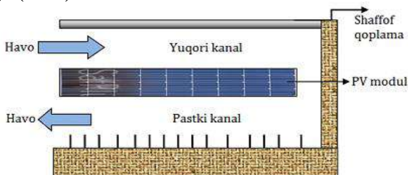
3-rasm. Pastki kanalida qovurg'a o'rnatilgan ikki yo'lli havoli PVT tizimi
