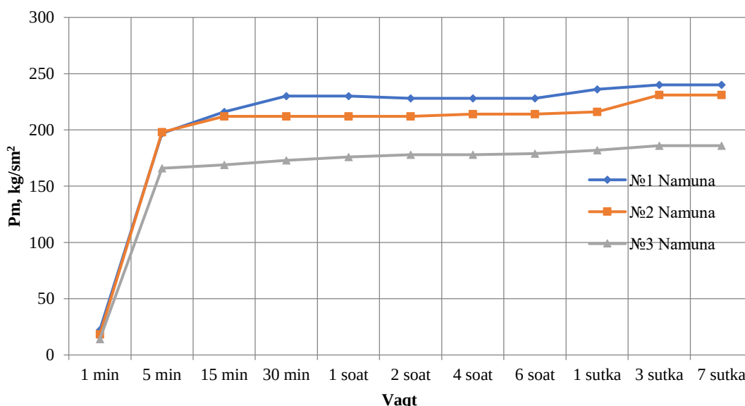
2 rasm. 300-320 ° C haroratda olingan gips bog'lovchilarining suspenziyalarida struktura hosil bo'lishining kinetikasi S/G 0,5
