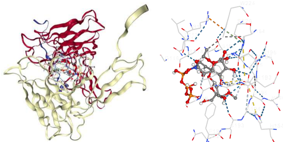
Рисунок 3. Молекулярная модель взаимодействия наноаскорбата хитозана с сульфатом алюминия с белком Pseudomonas aeruginosa .
