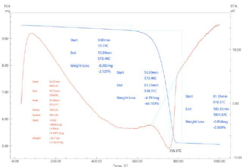
Рис.1–Дифференциально-термический анализ (ДТА) Джамансайского известняка.
