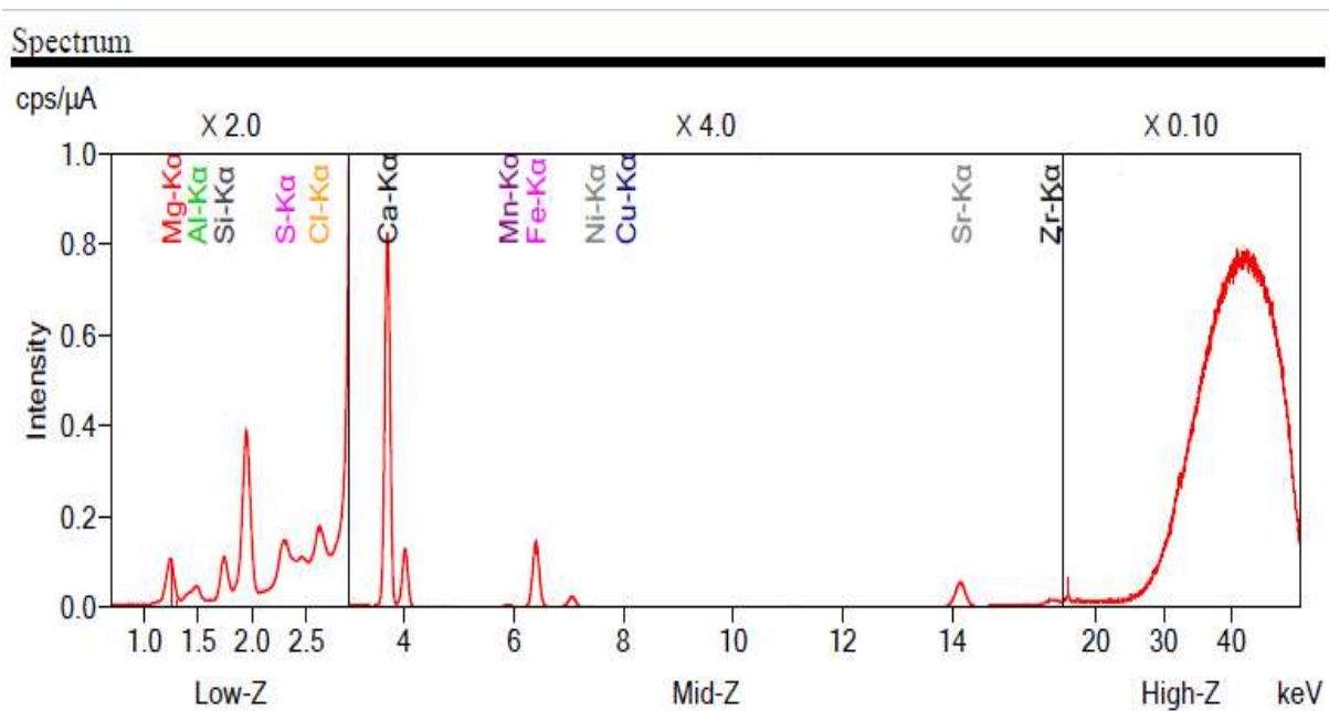
б) 1-расм. Жамансай хом доломитининг рентген-флуоресцент спектрлари. а) элементар; б) оксидли
