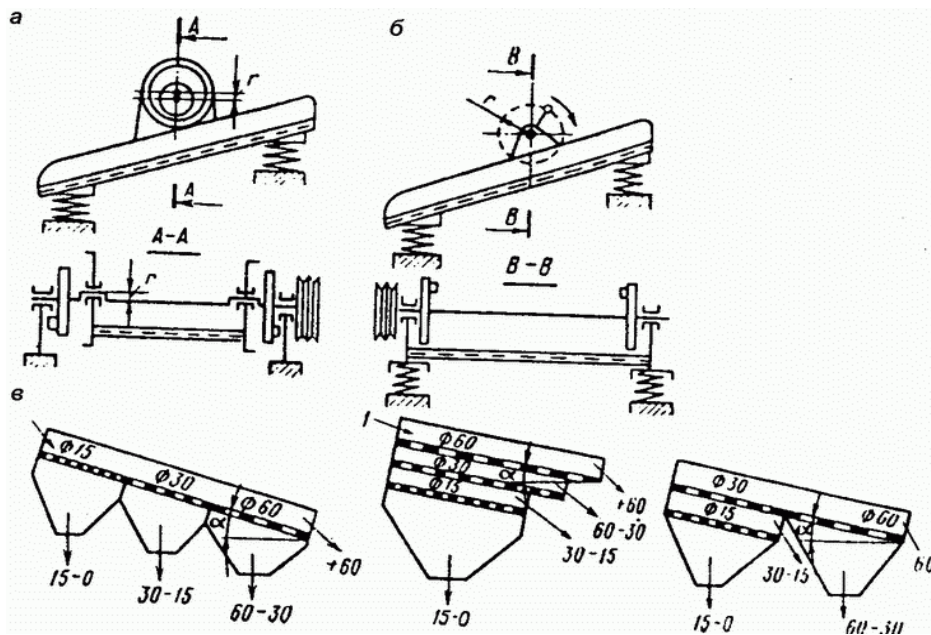
1- rasm. Tebranma g'alvirning tuzilish sxemasi.
