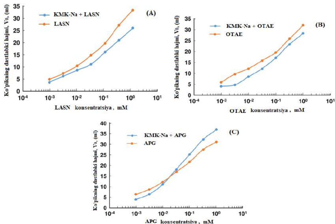
1-rasm. Karboksimetilkraxmal - sirt faol moddalar tizimlarining ko'pik hosil qilish qobiliyatiga sirt faol modda konsentratsiyasiga bog'liqligi. KMK-Na ning konsentratsiyasi 0,30 %.
