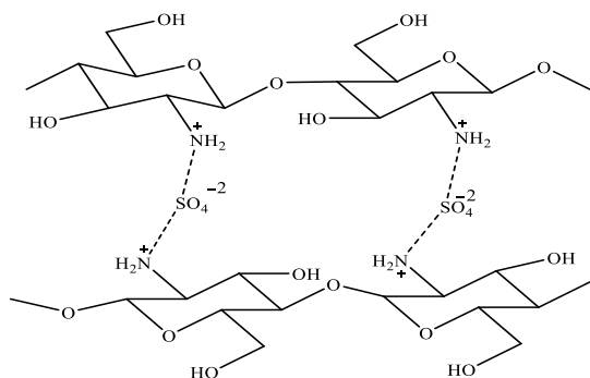
Рисунок 1. Сшивка сульфат-анионами макромолекул хитозана
