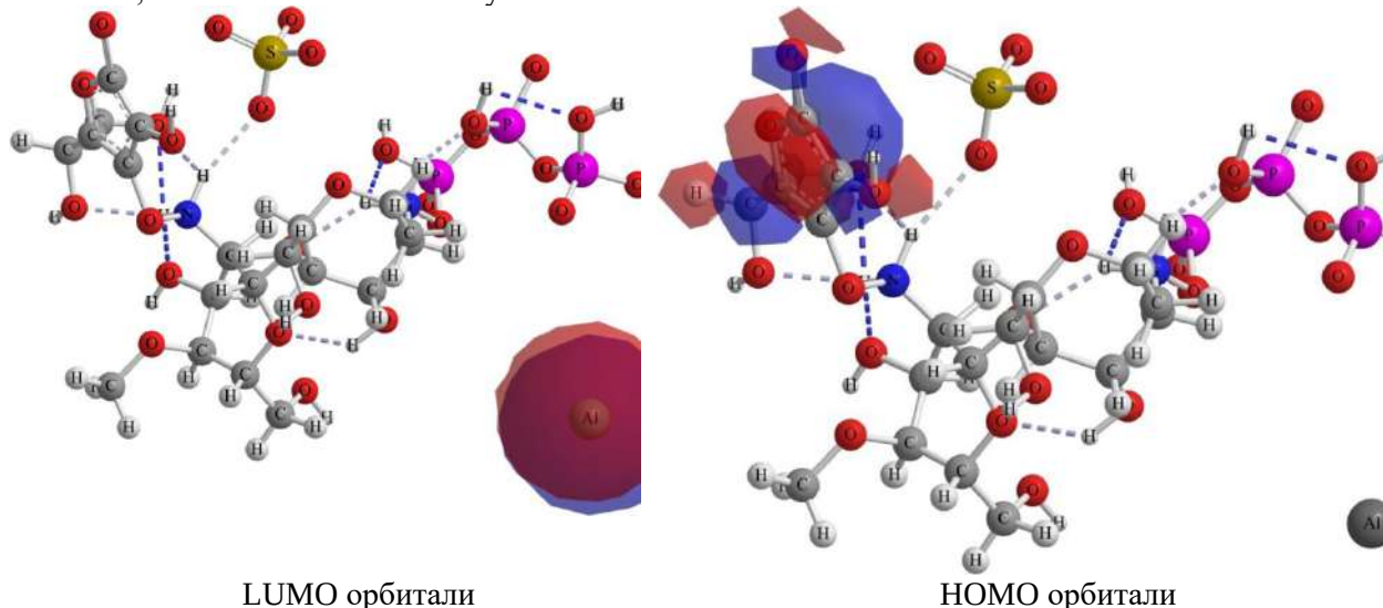
Рисунок 2. Граничные молекулярные орбитали исследованной системы.
