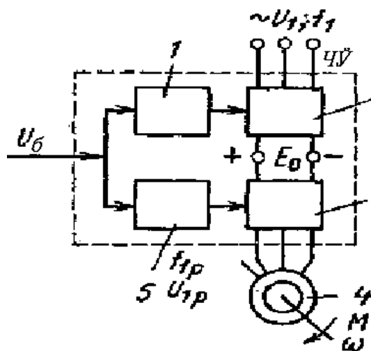
3 – расм. Ўзгармас ток бўғинли частота ўзгарткичнинг схемаси
