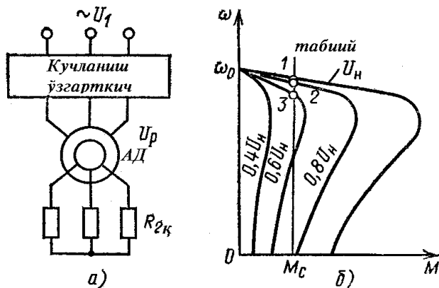
4-расм. АД координаталарини статордаги кучланишни ўзгартириш орқали ростлаш: а – схема; б - механик характеристикалар
