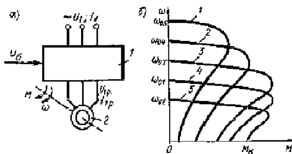
1-расм. Частотавий ростланадиган асинхрон электр юритманинг схемаси (а) ва механик характеристикалари (б)
