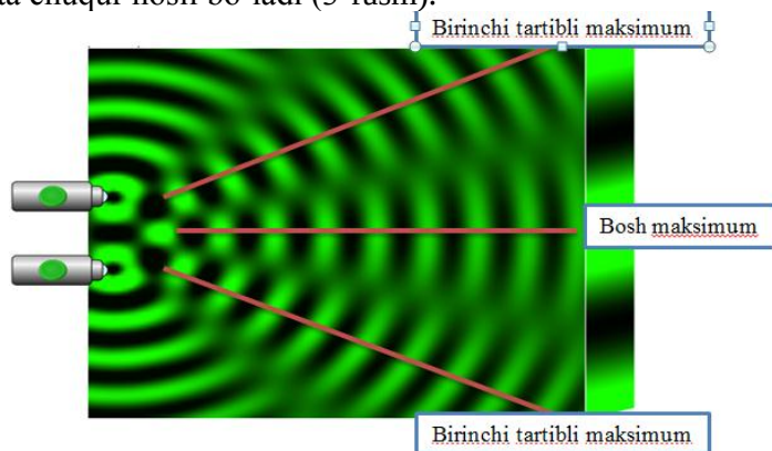
2-rasm: Kogerent to'lqinlar uchrashganda hosil bo'ldigan maksimumlar (do'ngliklar).
