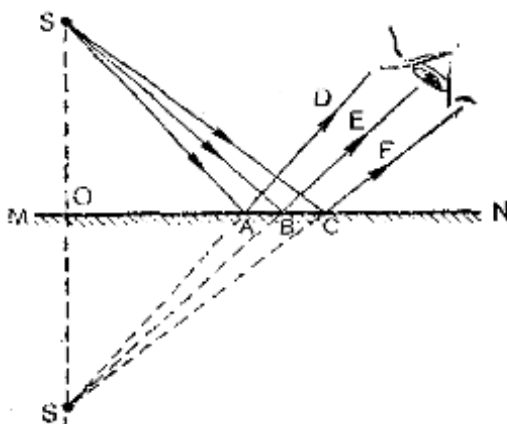
3-rasm. Yassi ko'zguda nuqta mavhum tasvirining hosil bo'lishi.
