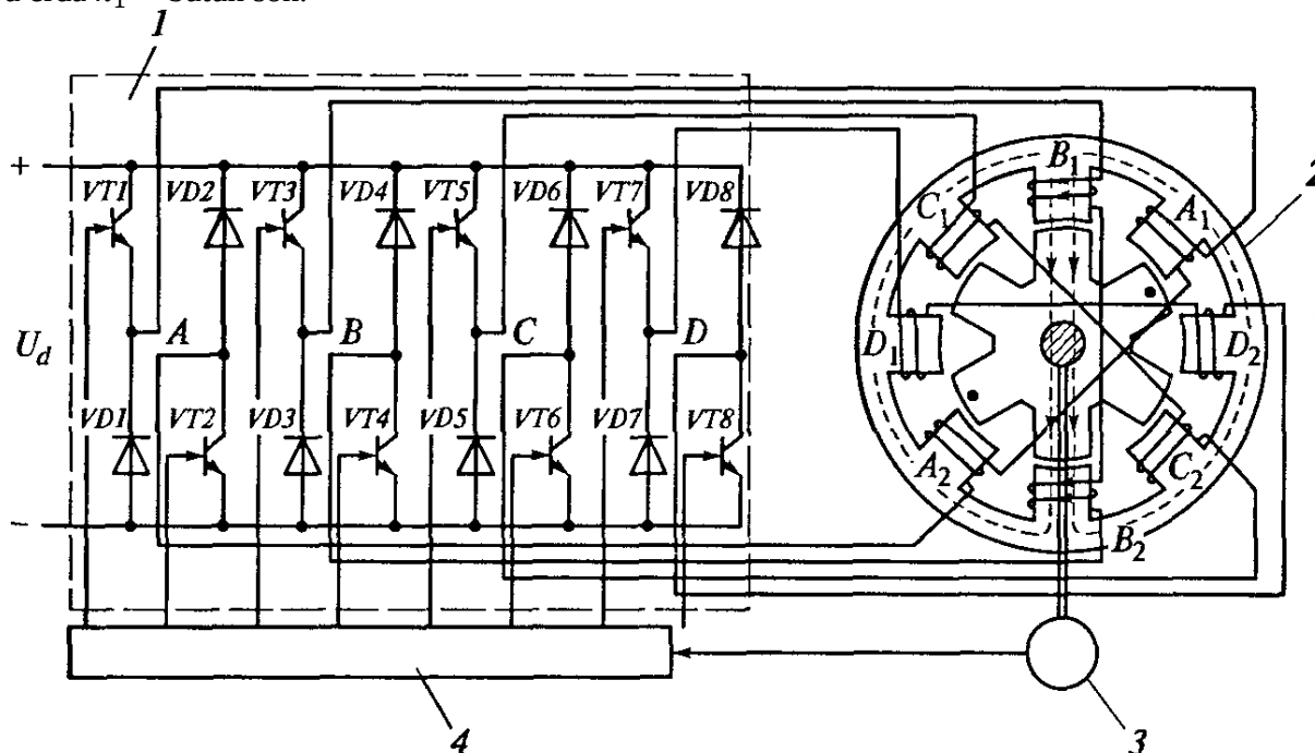
1-rasm. Ventelli-induktorli dvigatelning tuzilmasi:
