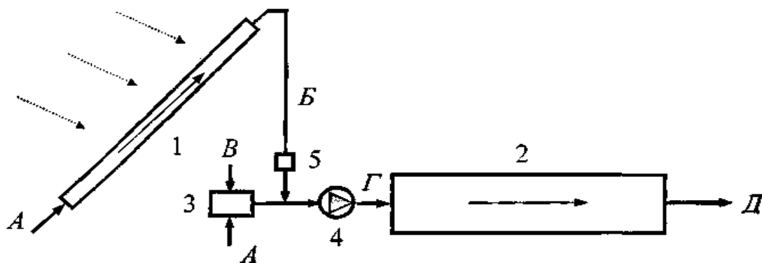
1-rasm. Kombinatsiyalashgan quyosh-yoqilg'i issiqlik manbali baraban tipli quritish qurilmasi texnologik sxemasi:
