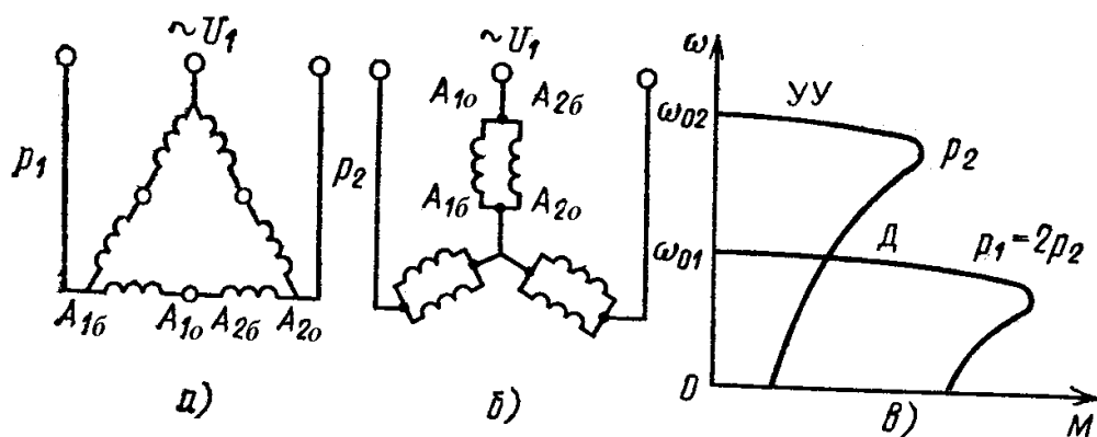
2-расм. АД статор чўлғамларини «учбурчак» (а), «иккиланган юлдуз» (б) кўринишида улаш ва учбурчак - иккиланган юлдуз схемаларининг механик характеристикалари (в).
