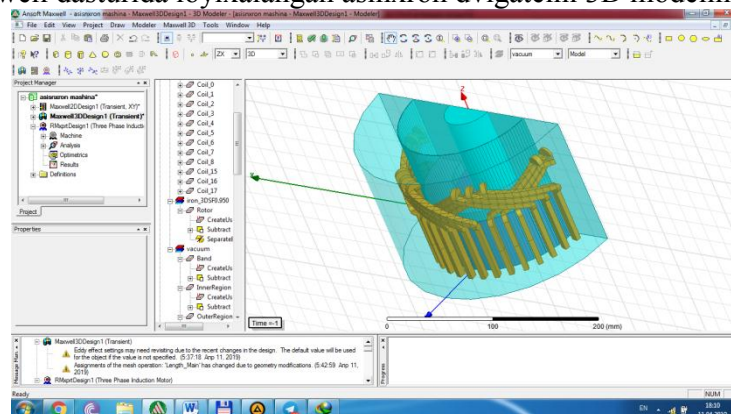
4-rasm.Maxwell dasturida loyixalangan asinxron dvigatelni 3D modelini ko'rinishi.
