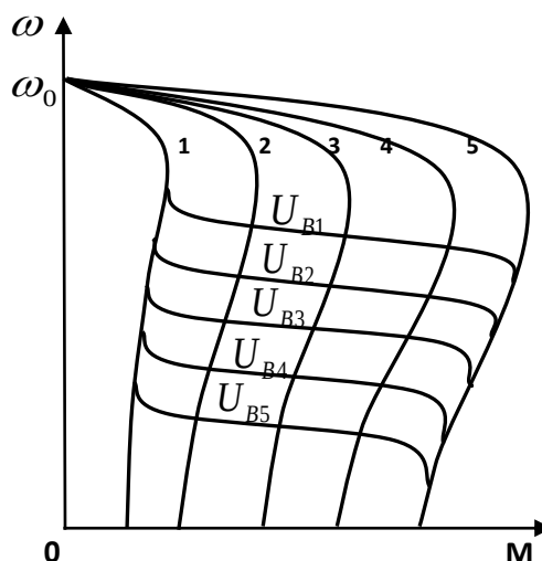
2 – расм. ТКРлиавтоматлаштирилганасинхронэлектрюритманинг механик тавсифлари.
