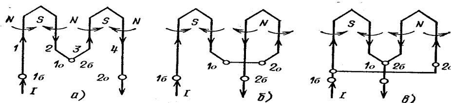
1-расм. АД статор чўлғамларининг жуфт кутбларисони ўзгартириш
