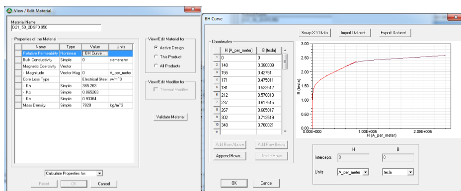
1-rasm. D21_50_2DSF0.950 tipidagi metallning xususiyatlari
