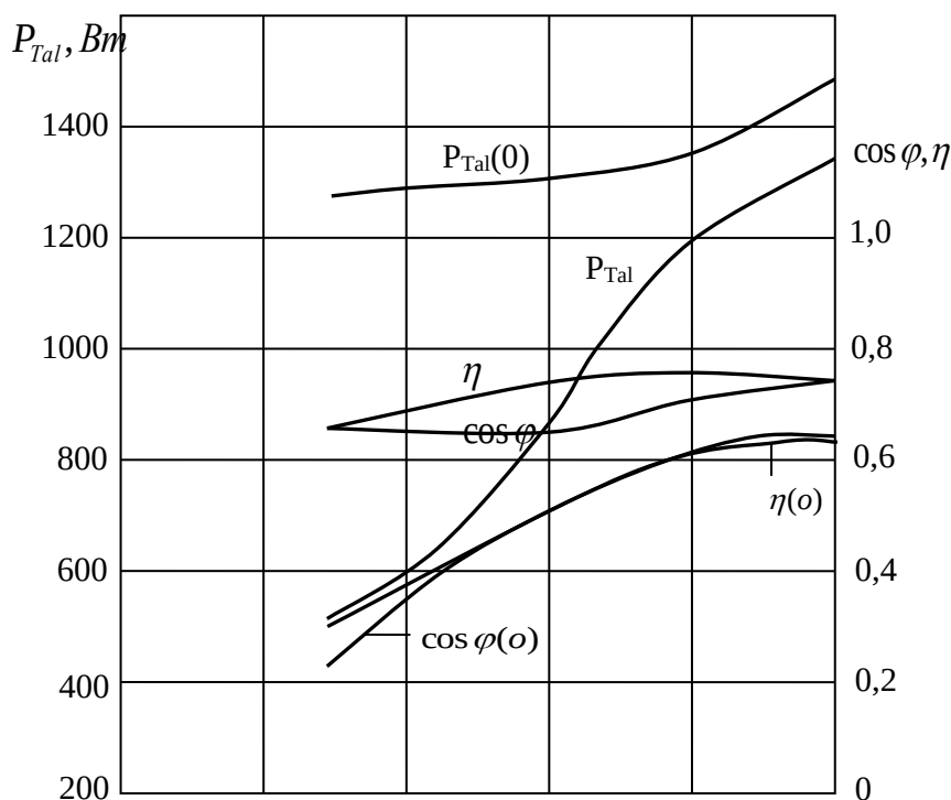
3 -расм. Контроллерли энергия тежамкорасинхронэлектрюритманинг ишчи тавсифлари .
