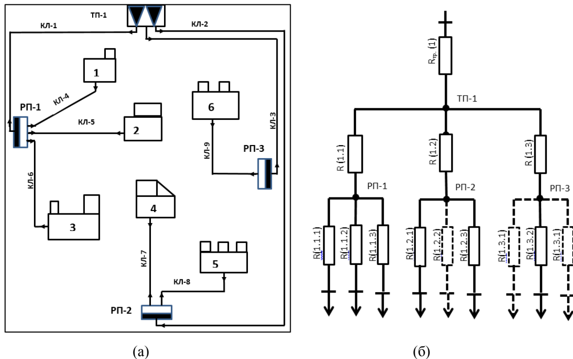
Рис.1. Схема электроснабжения -(а) производственного цеха и расчетная схема -(б) для составления матрицы исходных данных.
