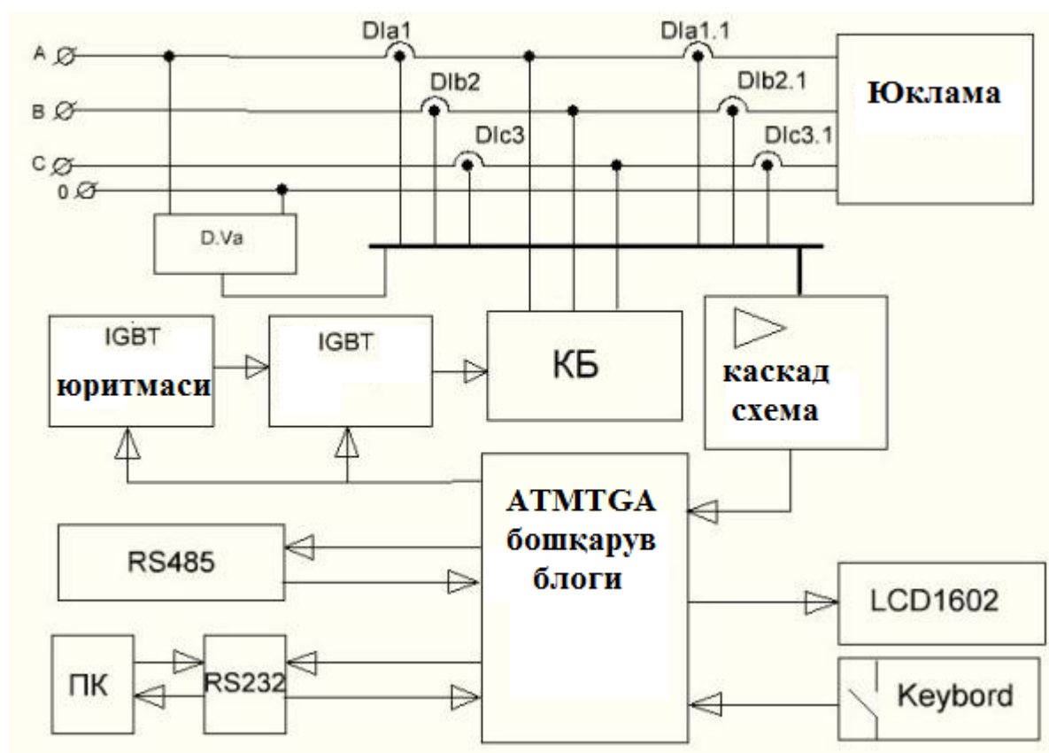
2-расм. Реактив қувват компенсацияси учун микроконтролерни бошқариш тизимининг блок схемаси.
