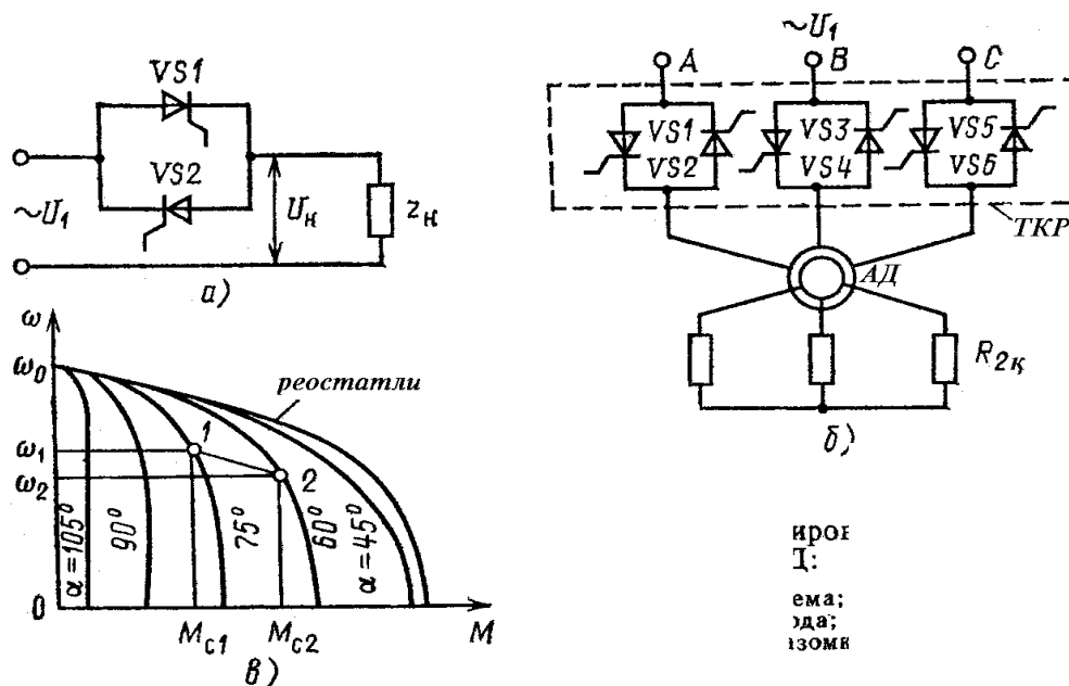
4-расм. «ТКР-АД» тизимида координаталарни ростлаш: а – бир фазали схема; б – электр юритманинг очик схемаси; в – очик схеманинг механик характеристикалари
