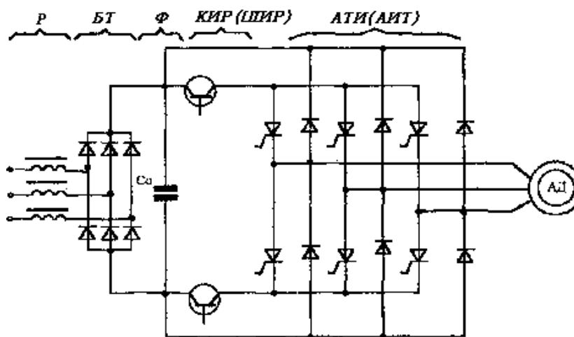
4 – расм. Частота ўзгарткичнинг комбинациялашган схемаси: P – индуктивли реактор; BT – бошқарилувчи тўғрилагич; Φ –сигимли филтр; KIP – кучланишнинг импульс ростлагичи; АТИ –автоном ток инвертори
