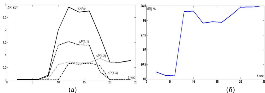
Рис.3. Кривые изменения потерь КЛ и суммарные потери КЛ подключенных к ТП - (а) и КПД электропотребления цеха (б).
