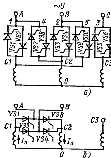
5-расм. ТКР дан АД ни тескари айлантириш (а) ва динамик тўхтатиш (б) учун фойдаланиш
