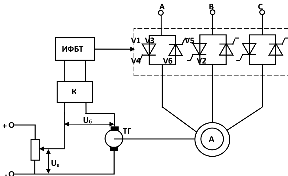
1 – расм. ТКРлиавтоматлаштирилганасинхронэлектрюритманинг функционал схемаси.
