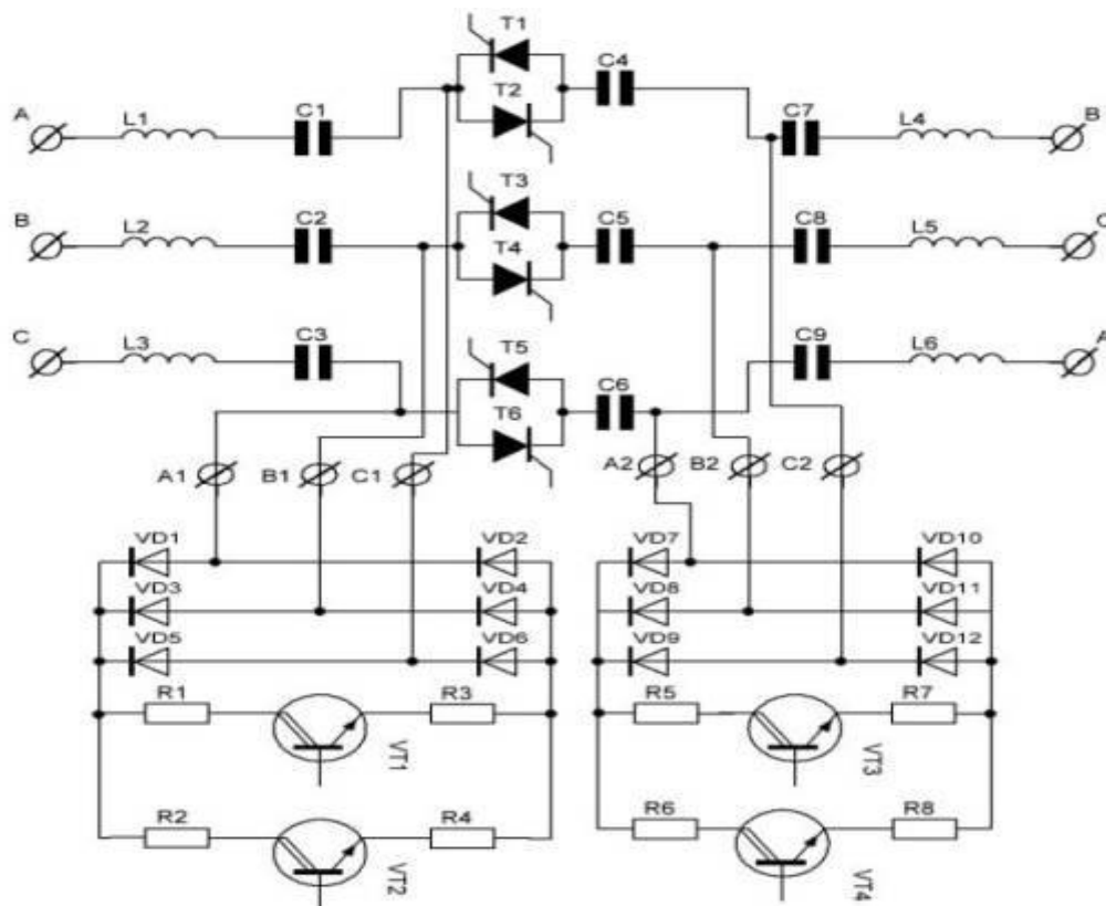
1-расм. Олтига тезликли реактив қувват компенсаторининг кучланиш ўчириш диаграммаси
