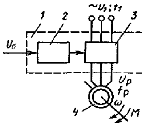
2- расм.Бевосита боғла-нишли частота ўзгарткичнинг блок-схемаси
