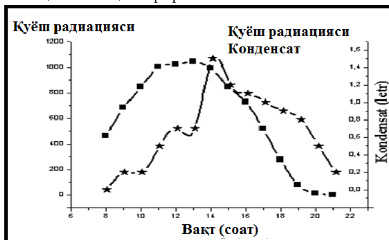
2-график. Энергетик такомиллашган парник типли қуёш сув чучутгичига тушаётган қуёш радиацияси ва олинган конденсатнинг вақтга боғлиқлик графиги.
