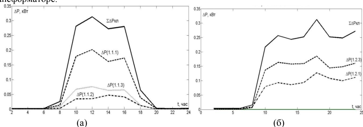
Рис.2. Кривые изменения потерь КЛ и суммарные потери КЛ подключенных к РП-1(а) и РП-2 (б).
