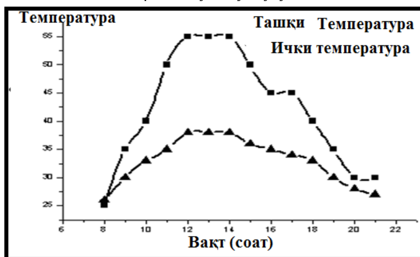
1-график. Энергетик такомиллашган парник типли қуёш сув чучутгичининг ички ва ташқи температуранинг вақтга боғлиқлик графиги.
