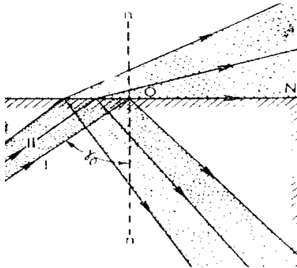
4b- rasm. I nur shisha—havo chegarasi bo'ylab ketadi
