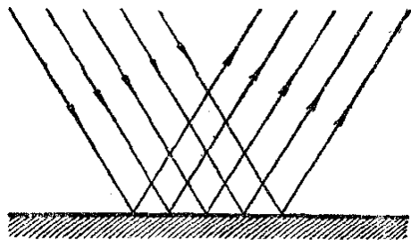
2 -rasm. Yorug'likning tekis sirtidan qaytishi.
