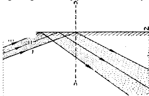
4v- rasm. Yorug'lik nurlarining tushayotgan butun dastasi shisha ichiga qaytadi.
