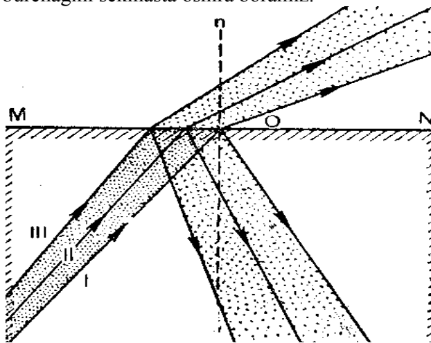
4a-rasm. Yorug'lik nurlarining tarqaluvchi dastasi shishadan havoga o'tadi.
