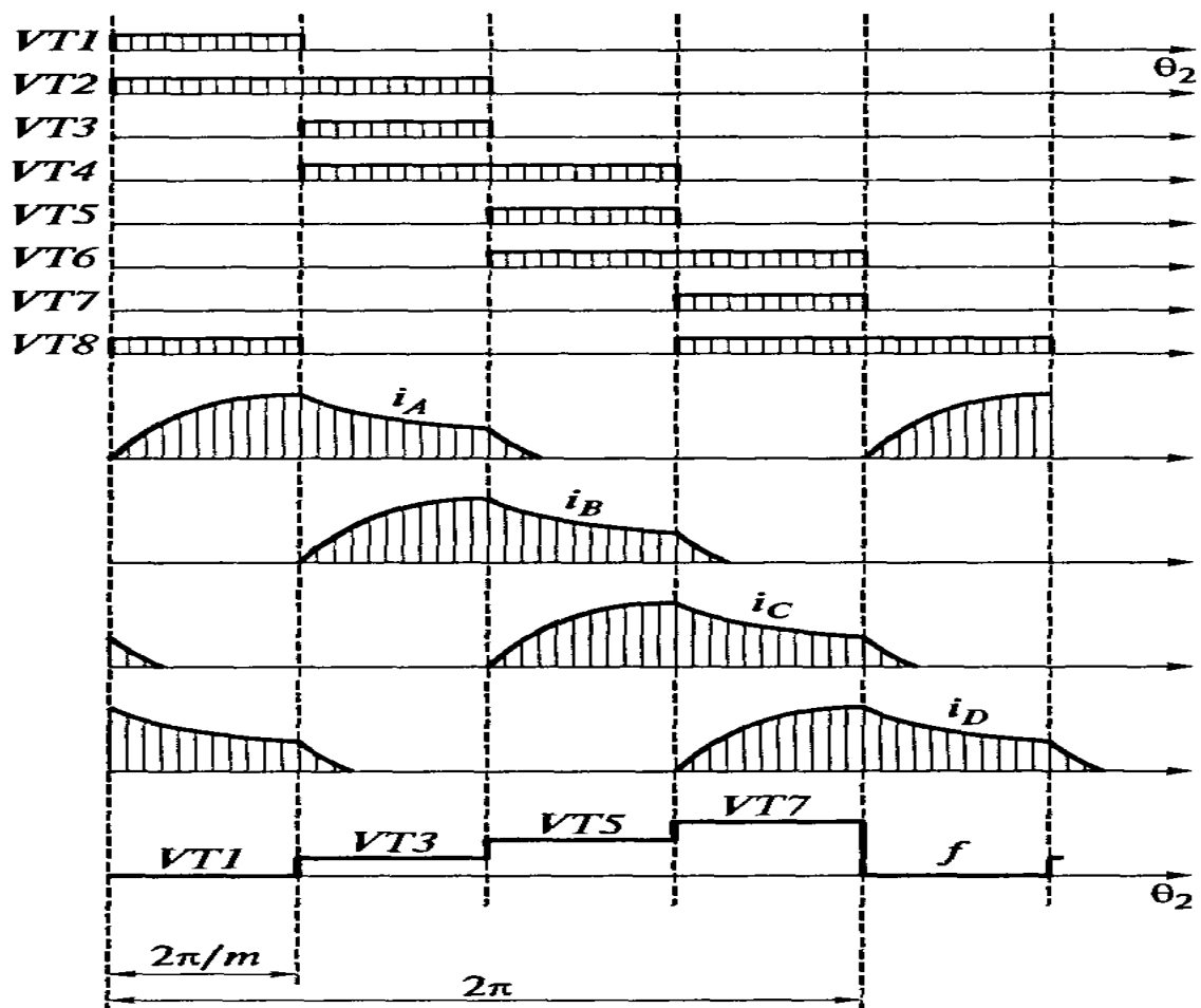
2-rasm. Ventil-induktorlidvigateľfazacho'lg'amlardagitoklarning shakllanishi.
