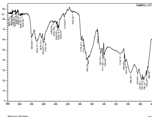
2-rasm. 1:3 molyar nisbatda sianur kislota va metafosfat kislotasi hosil qilgan birikmaning infraqizil (IQ) spektri.
