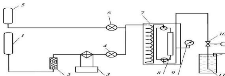
1- rasm. Dinamik eruvchanlikni o'lchash uchun eksperimental birlik (sxema); (1) CO 2 bilan silindr; (2) filtr namligini yo'q qiluvchi; (3) xolodilnik; (4), (6) nasoslar; (5) erituvchi bilan idish; (7) havo termostatni; (8) extractor; (9) manometr; (10) bosim nazoratchi; va (11) suv bilan idish
