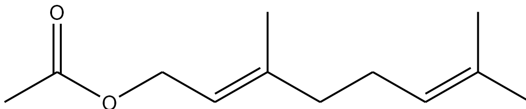
3,7-dimetyl-trans-2,6-octadien-1-ol asetat
