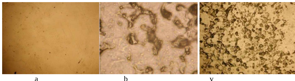
3-расм. Композициялар ОК (а), ОК-ГИПАН (б) ва ОК-КМС-На (в) тегишлича микрофотографиялари: а ва б – 100\times , в – 400\times марта катталаштирилган оптик суратлари.
