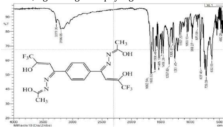
1-rasm. \text{H}_4\text{L}^1 ning IQ spektri va tuzilishi
