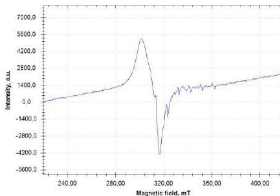
2-rasm. [CuL^1 \cdot 2L^2] kompleksning EPR spektri
