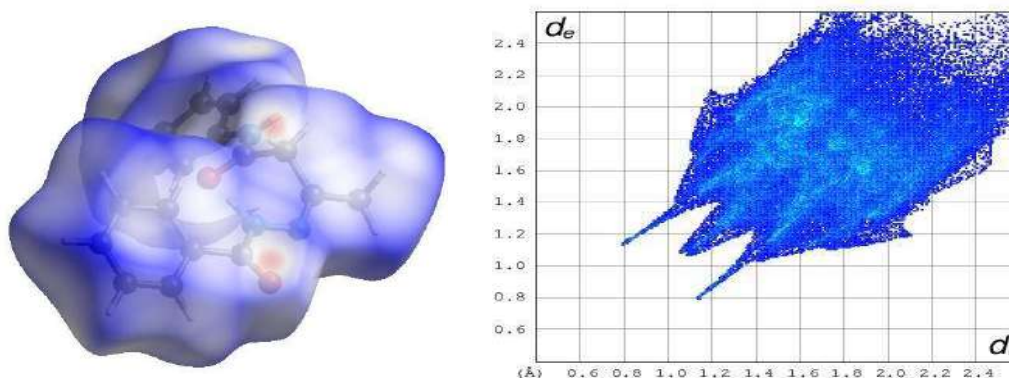
1-rasm. Neytral atsetoatsetanilid benzoilgidrazoni molekulasi d_{\text{norm}} (yuqori) va ikki o'lchovli barmoq izlari (pastki) bo'yicha tasvirlangan Hirshfeld sirtlari tasviri.
