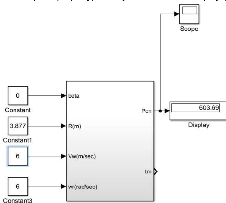
5-расм. Шамол параметрлари турлича бўлгандаги қийматлари учун натижа
