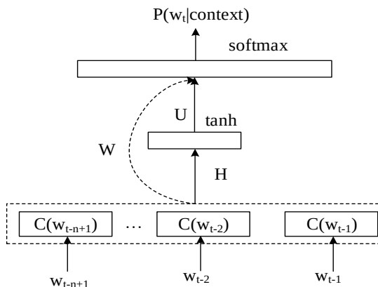
1-rasm. FFNN-til modeli arxitekturası
