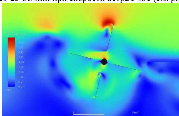
Рис. 3. Контур скорости V=5 \text{ м/с} .
