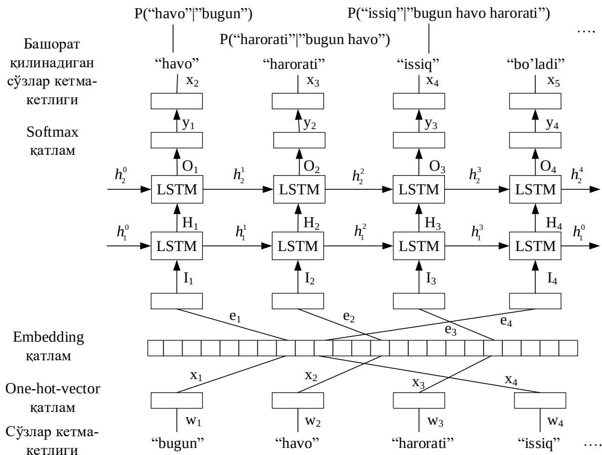
3-rasm. Neyron til modeli strukturasi
