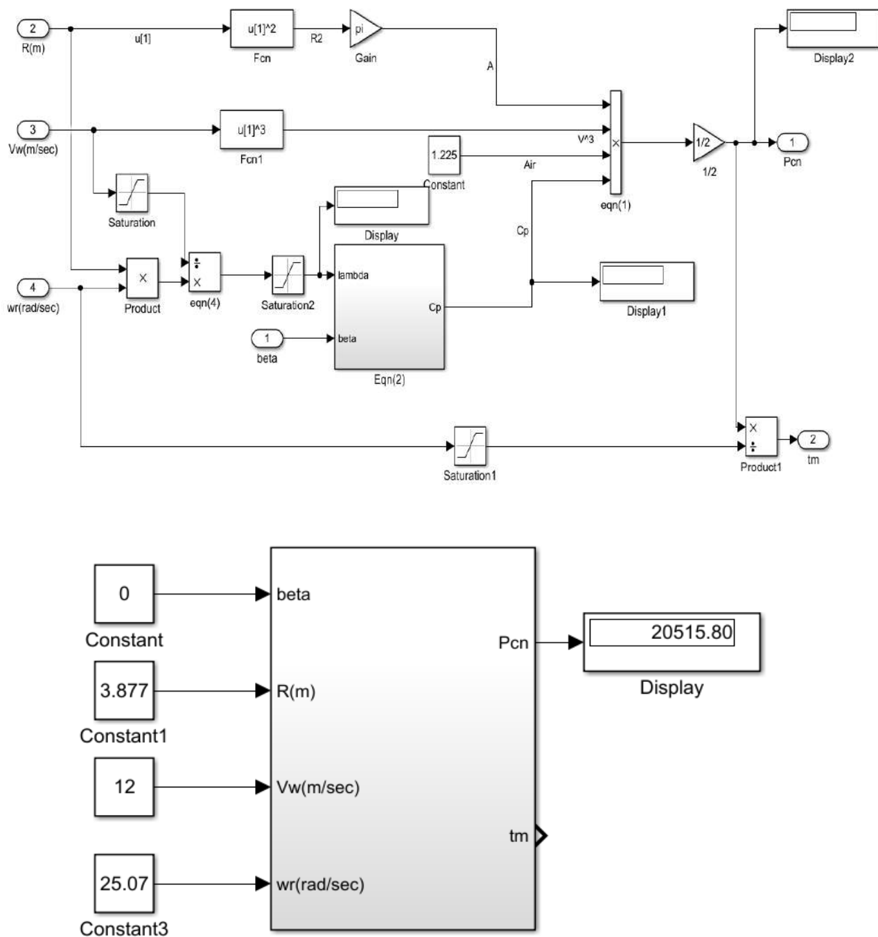
1-расм. Шамол турбинасининг математик модели.
