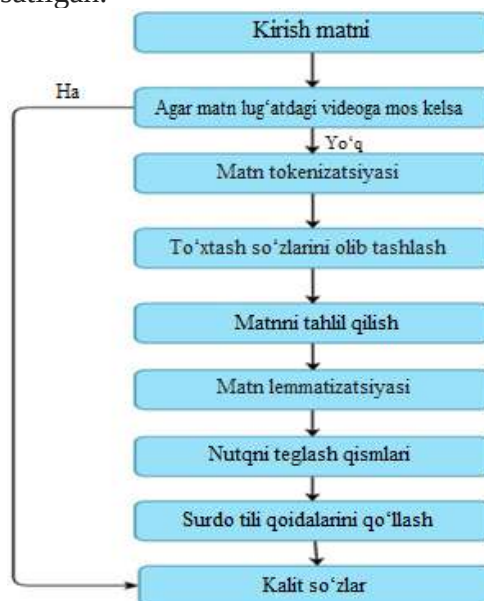
4-rasm. Tabiiy til modeli arxitekturasini.
