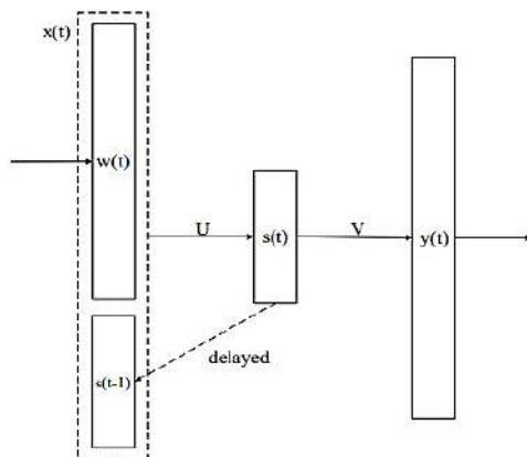
2-rasm. RNN- til modeli arxitekturası
