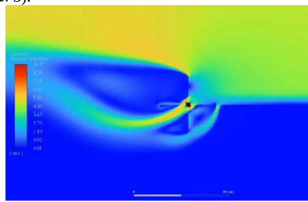
Рис. 4. Контур скорости V=6 \text{ м/с} .
