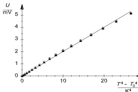
3-rasm. U chiqish kuchlanishining T^4 - T_0^4 funksiyasi sifatidagi grafigi.
