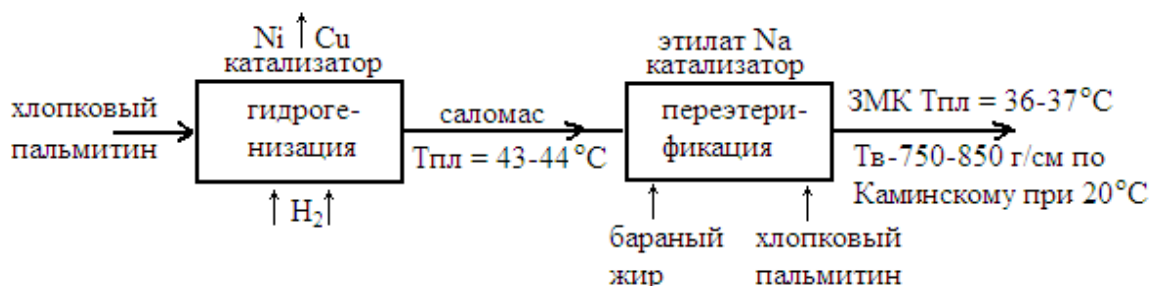
Рис.1. Блок-схема получения ЗМК путем гидрогенизации хлопкового пальмитина с последующей переэтерификацией полученного гидрогенизата с хлопковым пальмитином и животным (бараньим) жиром
