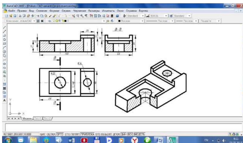
7-shakl. Qirqimning to'liq bajarilgani
