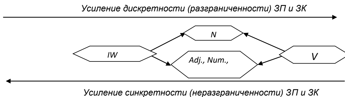
Рис. 2. Разграничение ЗП и ЗК лексико-семантическим способом**
