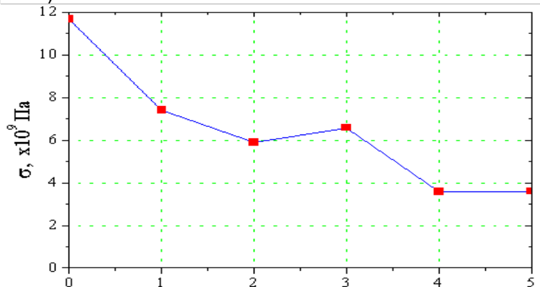
Таъсир қилиш вақти, с 1-расм. TiV_x - n - n^+GaAs структурасида ИМКнинг \sigma микротўлқинли таъсир вақтига боғланиши
