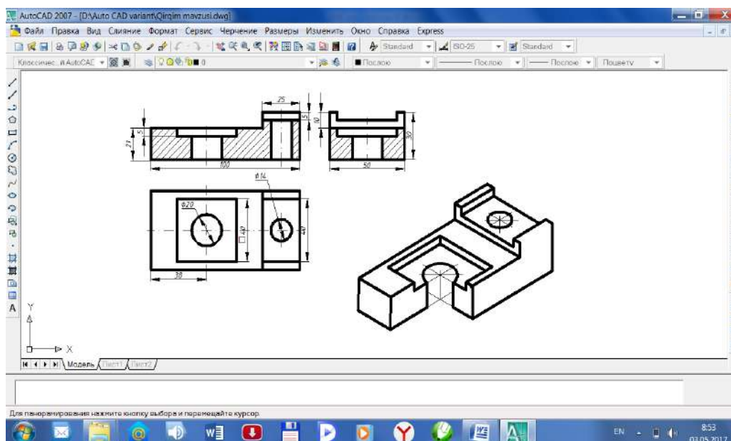
5-shakl. Yaqqol tasvirda yordamchi chiziqlar bo`ylab detalning yaqqol tasviridan to`rttdan bir qismini kesib olish
