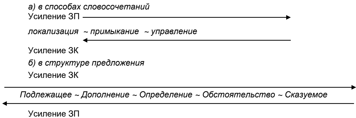
Рис. 4. Разграничение ЗП и ЗК
