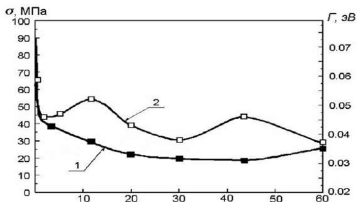
Нурланиш вақти, с 2-расм. Ички механик кучланиш \sigma нинг ва параметр кенгайиши \Gamma нинг микротўлқин вақтига боғлиқ ўзгариши
