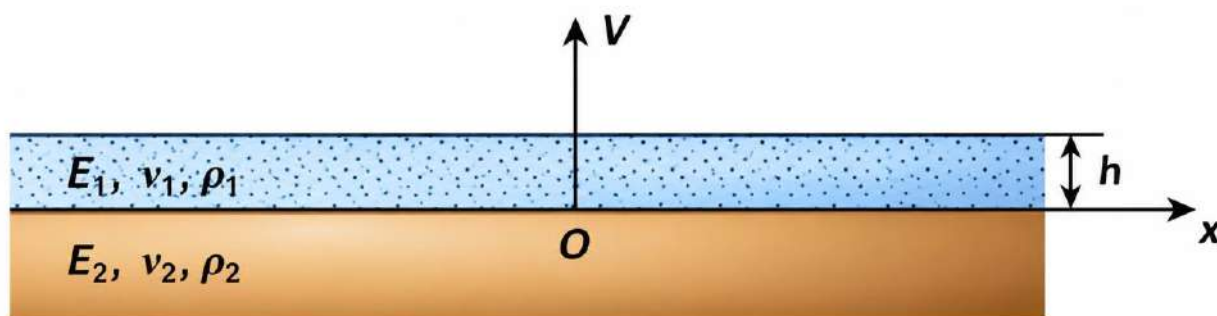
Рисунок 1. Расчетная схема системы «вязкоупругий слой – вязкоупругое полупространство».
