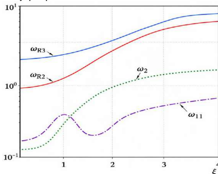
Рисунок 3. Комплексный спектр собственных частот диссипативно неоднородной системы
