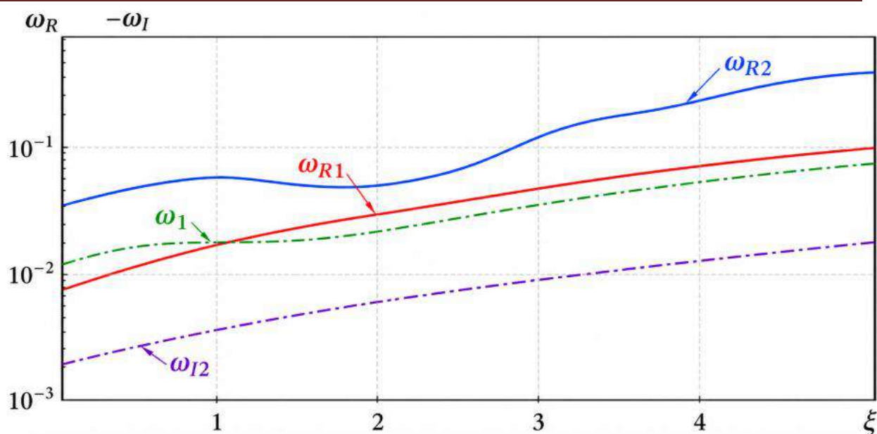
Рисунок 4. Комплексные собственные частоты от безразмерного волнового числа \xi при скользящем контакте: диссипативно однородная система
