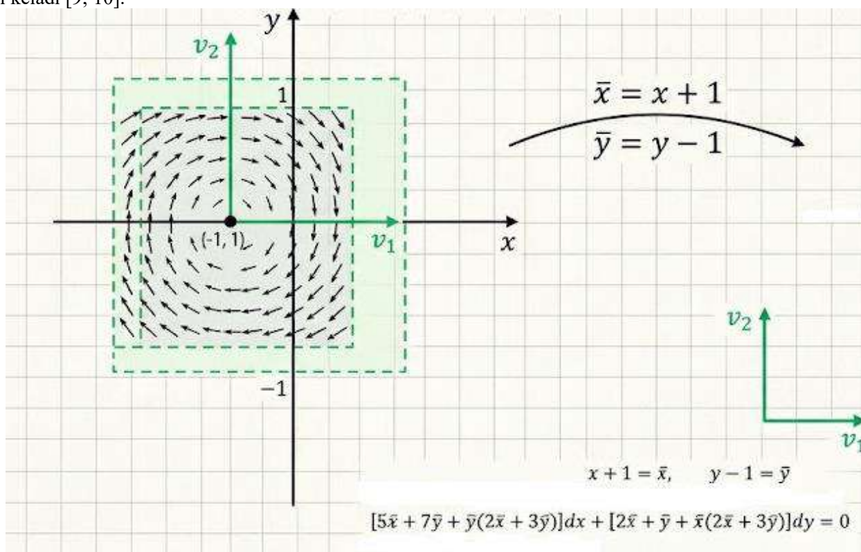
1-rasm. Darbu tenglamasining geometrik interpretatsiyasi
