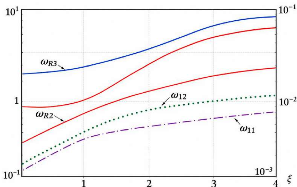
Рисунок 2. Зависимость комплексных собственных частот от безразмерного волнового числа \zeta для диссипативно однородной системы
