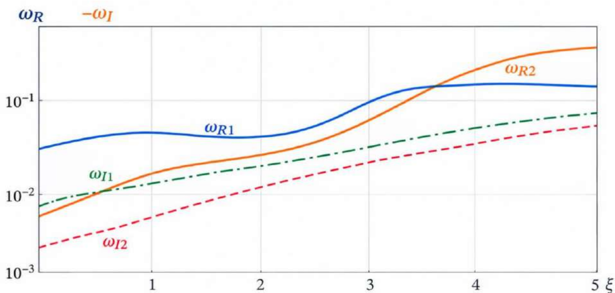
Рисунок 5. Комплексные собственные частоты от безразмерного волнового числа \xi при скользящем контакте: диссипативно неоднородная система
