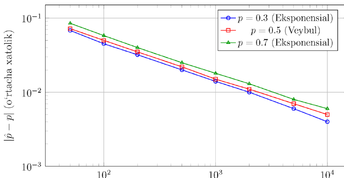
1-rasm. 10000 takrorlash bo'yicha o'rtacha xatolik |\hat{p} - p| ning tanlanma hajmiga bog'liq holda yaqinlashuvi
