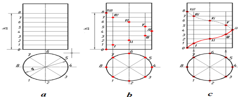
4-шакл. AutoCAD дастуридавинт чизиқ чизмасини бажариши босқичи
