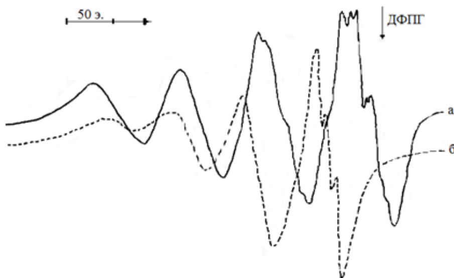
Рис. 4. Спектр ЭПР комплексного соединения \text{CuL}^{14} \cdot \text{NH}_3 в растворе хлороформа–(а) и \text{CuL}^{16} \cdot \text{NH}_3 в растворе пиридина–(б) при 298 К.
