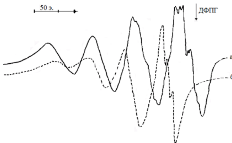
4-расм. CuL 14 ·NH 3 комплекс бирикманинг хлороформдаги – (а) ва CuL 16 ·NH 3 нинг пиридиндаги– (б) 298 К да олинган ЭПР спектрлари.
