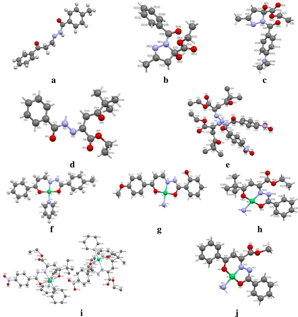
1-расм. Молекуляр структуралар: H_2L^8 -а, H_2L^{11} -б, H_2L^{13} -с, H_2L^{21} -д, H_2L^{23} -е, NiL^8 \cdot Py -ф, NiL^{10} \cdot NH_3 -г, NiL^{21} \cdot NH_3 -ҳ, NiL^{23} \cdot 3Py -и, NiL^{24} \cdot NH_3 -ж.
