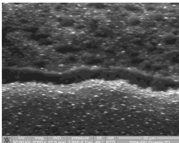
2 – rasm. \text{YBa}_2\text{Cu}_3\text{O}_{7-x} plyonkasining nurlangan va nurlanmagan hududlari orasidagi interfeysning skanerli elektron mikroskopiya tasviri
